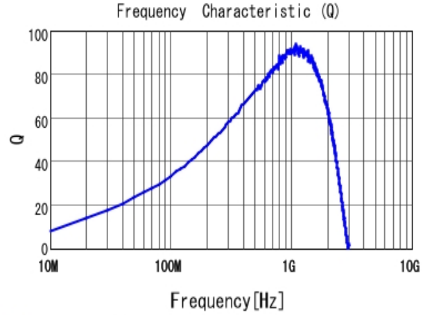
■ LQW2BAS24NJ00 Q
