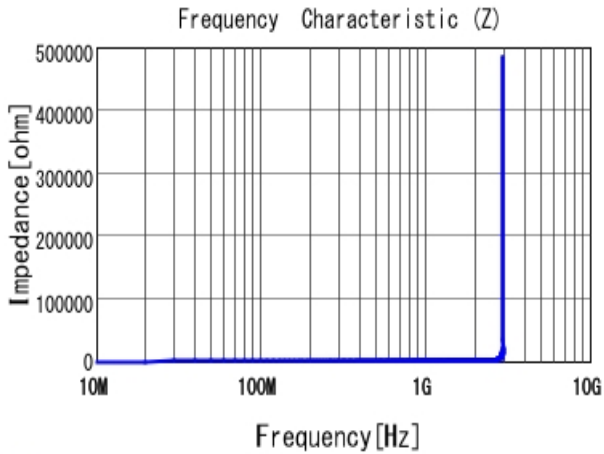
■ LQW2BAS24NJ00 |Z|
