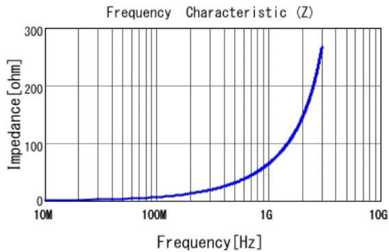
■ LQW2BAS10NJ00 |Z|
