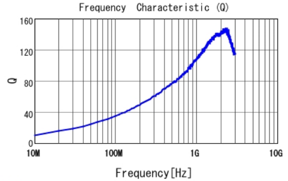
■ LQW2BAS10NJ00 Q
