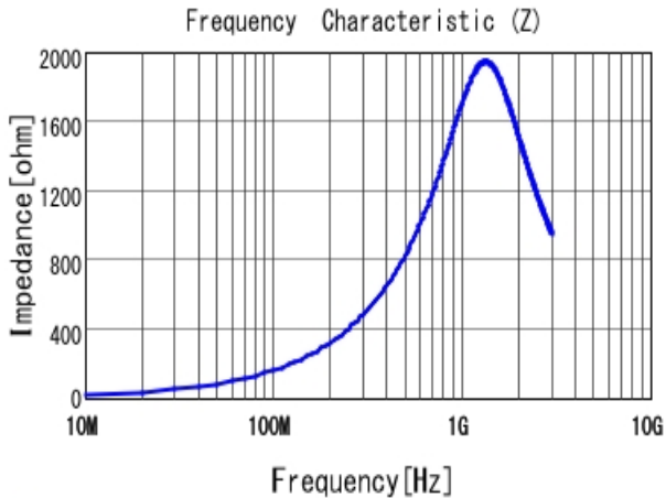
■ LQW18CNR27J00 |Z|
