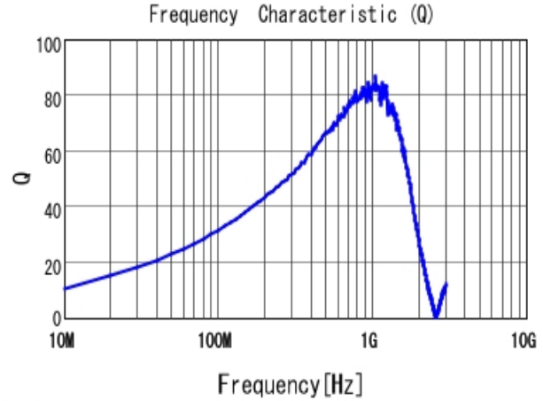
■ LQW18AN68NJ00 Q
