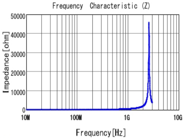
■ LQW18AN68NJ00 |Z|
