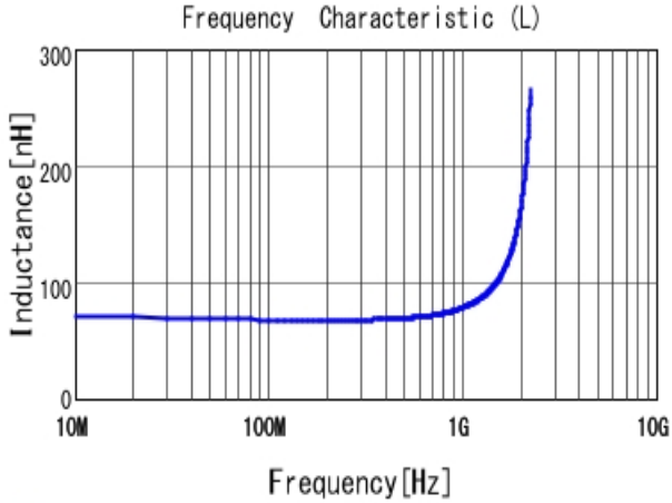
■ LQW18AN68NJ00 L
