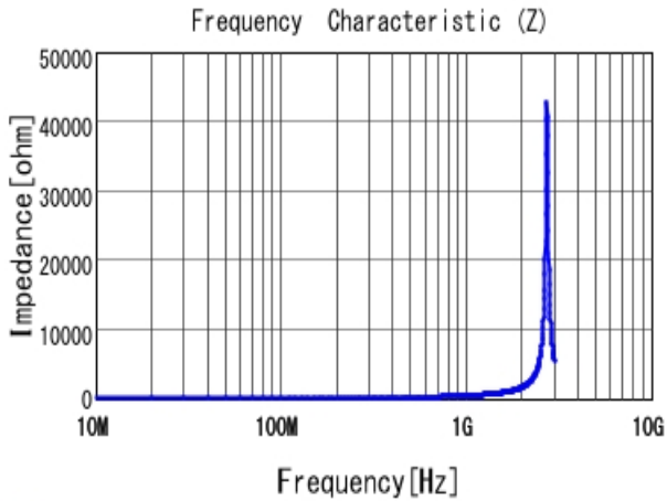
■ LQW18AN62NG00 |Z|
