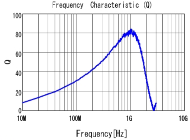
■ LQW18AN62NG00 Q
