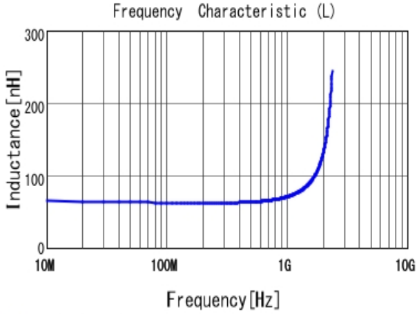
■ LQW18AN62NG00 L
