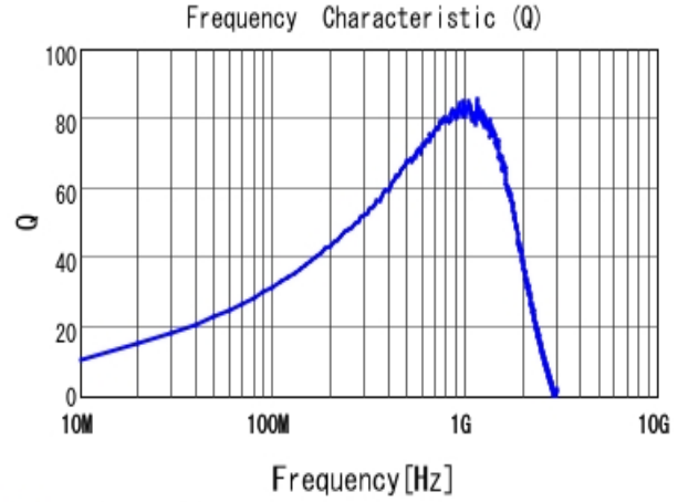
■ LQW18AN51NJ00 Q
