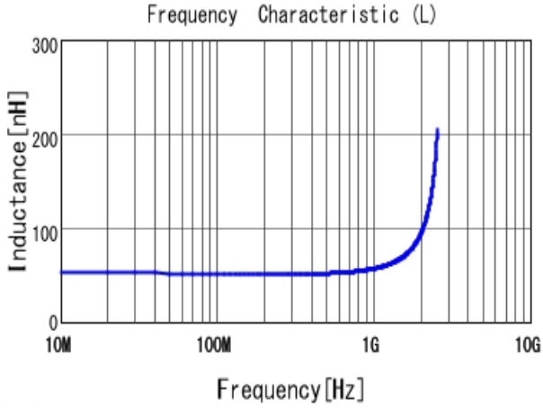
■ LQW18AN51NJ00 L
