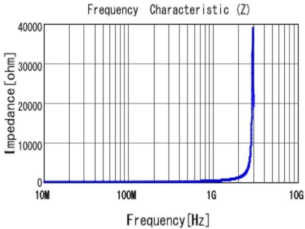
■ LQW18AN51NJ00 |Z|
