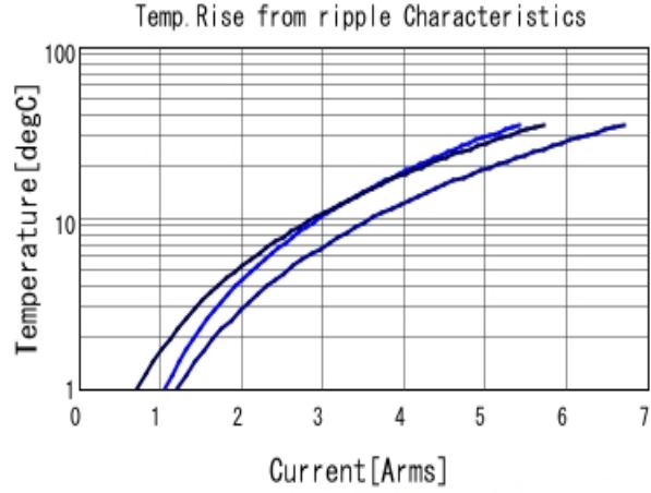
GRM32DR61C106KA01 Temp. rise ■ 80kHz ■ 400kHz ■ 800kHz
