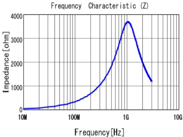
■ LQW18CNR56J00 |Z|
