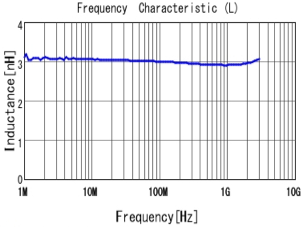
■ LQW18AN3N0C80 L
