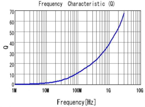
■ LQW18AN3N0C80 Q
