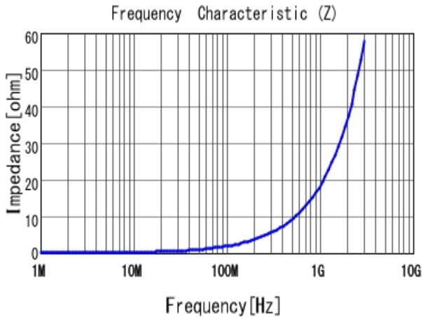
■ LQW18AN3N0C80 |Z|
