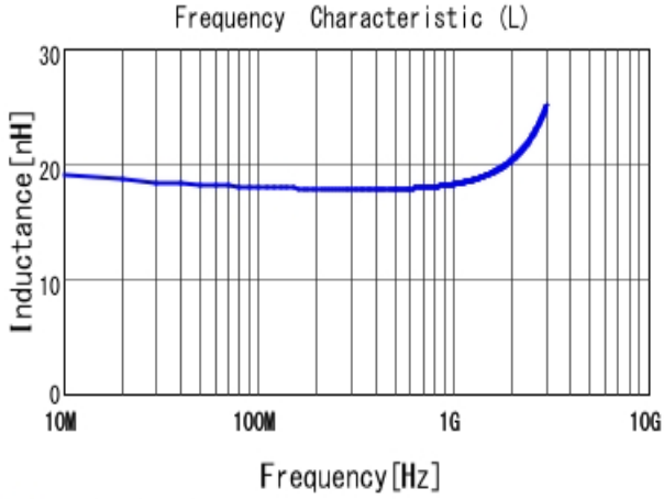
■ LQW18AN18NG10 L
