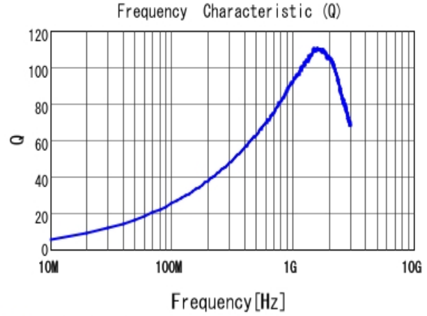
■ LQW18AN18NG10 Q
