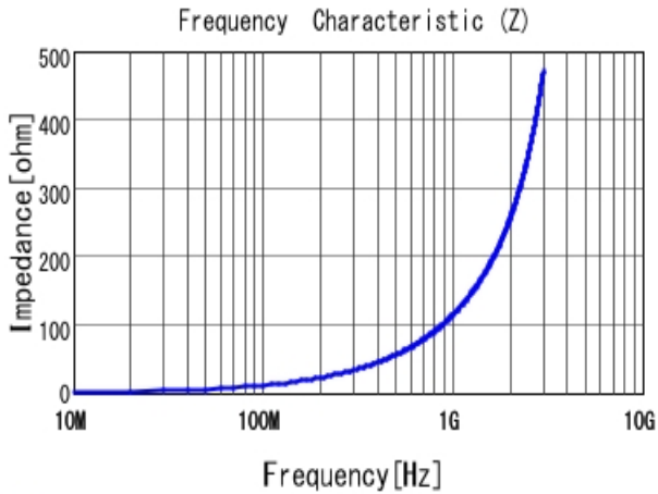
■ LQW18AN18NG10 |Z|
