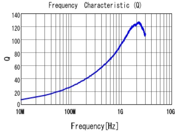
■ LQW18AN10NG10 Q
