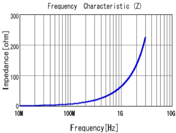
■ LQW18AN10NG10 |Z|
