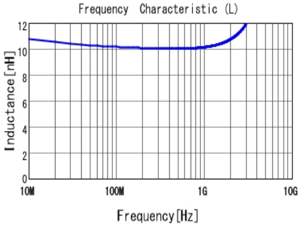
■ LQW18AN10NG10 L
