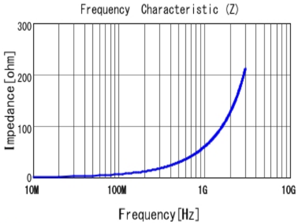
■ LQW15AN9N5G00 |Z|
