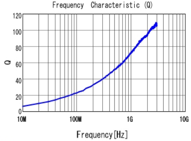
■ LQW15AN9N5G00 Q
