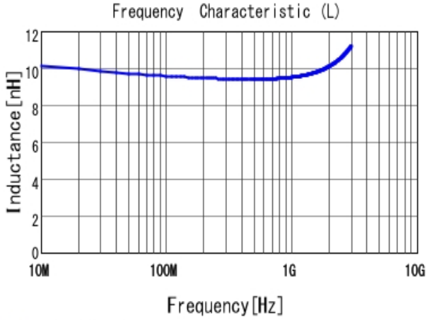
■ LQW15AN9N5G00 L
