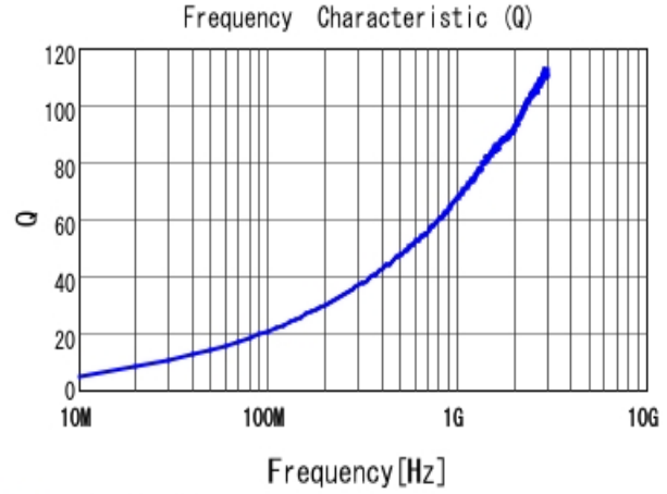
■ LQW15AN8N7H00 Q
