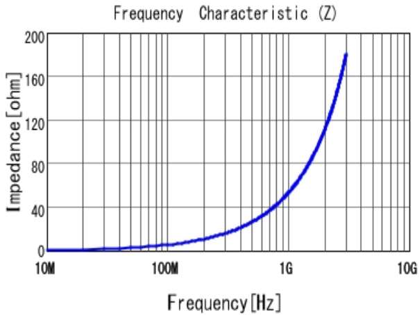
■ LQW15AN8N7H00 |Z|
