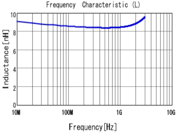
■ LQW15AN8N7H00 L
