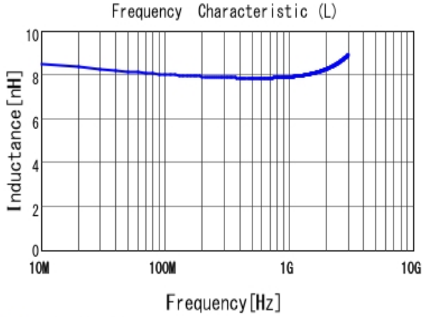
■ LQW15AN8N2J00 L
