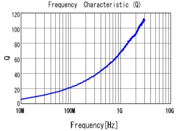
■ LQW15AN8N2J00 Q
