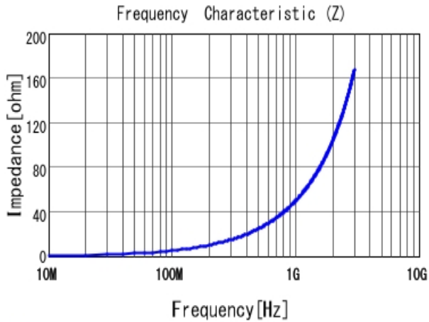
■ LQW15AN8N2J00 |Z|
