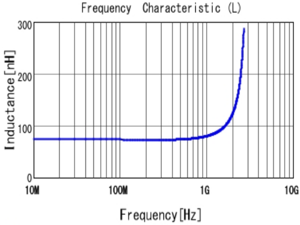
■ LQW15AN72NG00 L
