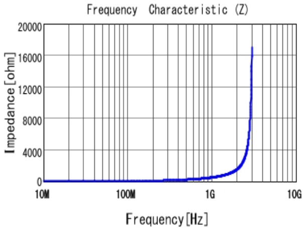
■ LQW15AN72NG00 |Z|
