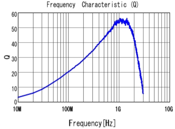
■ LQW15AN72NG00 Q
