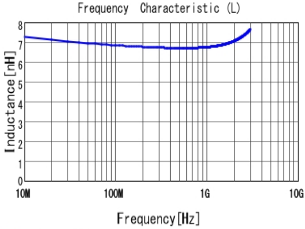
■ LQW15AN6N8H00 L
