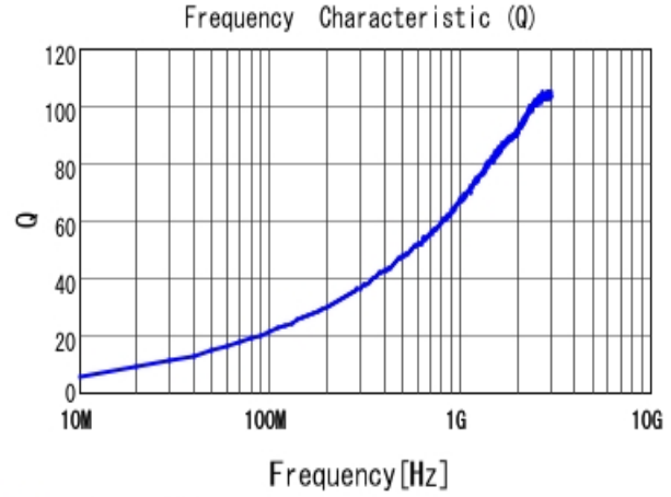
■ LQW15AN6N8H00 Q
