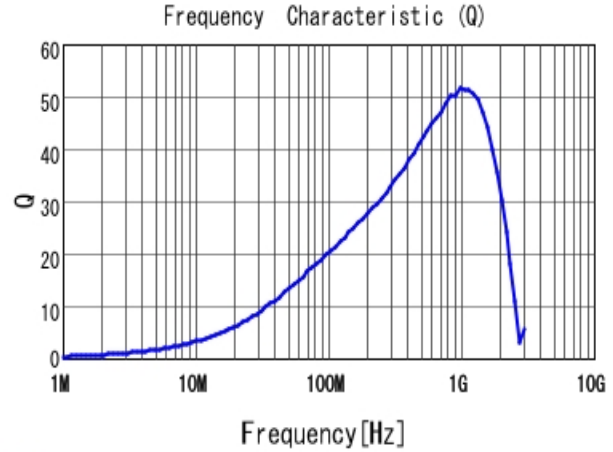
■ LQW15AN68NG80 Q
