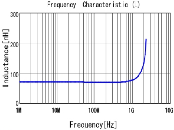
■ LQW15AN68NG80 L
