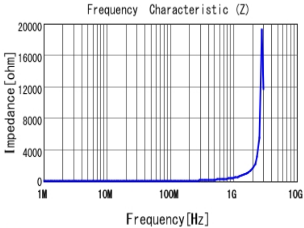
■ LQW15AN68NG80 |Z|
