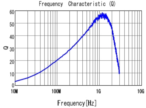
■ LQW15AN68NG00 Q
