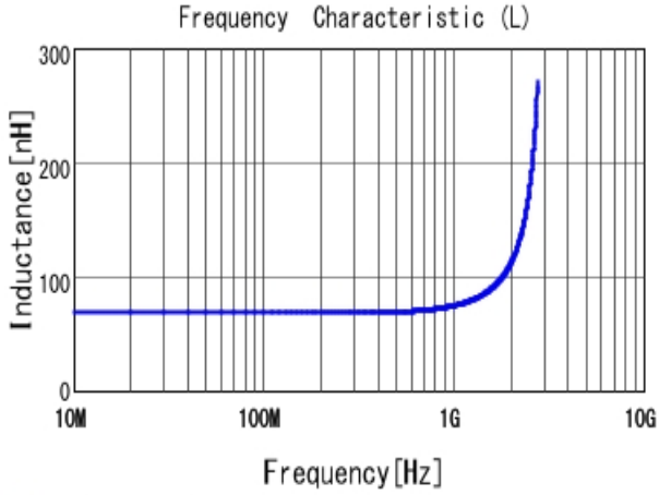
■ LQW15AN68NG00 L
