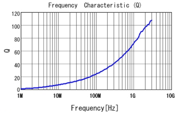
■ LQW15AN5N6B80 Q
