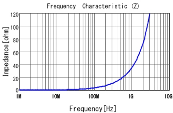
■ LQW15AN5N6B80 |Z|
