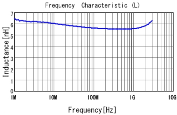
■ LQW15AN5N6B80 L
