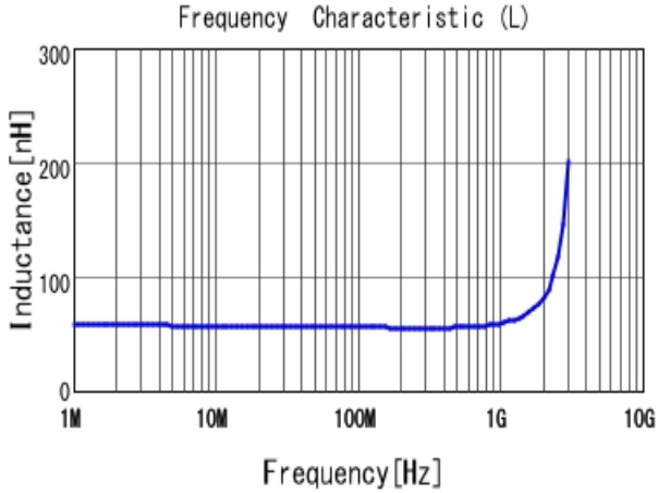
■ LQW15AN56NG80 L
