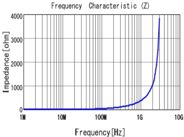
■ LQW15AN56NG80 |Z|
