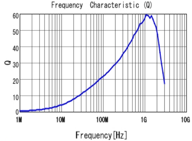
■ LQW15AN56NG80 Q
