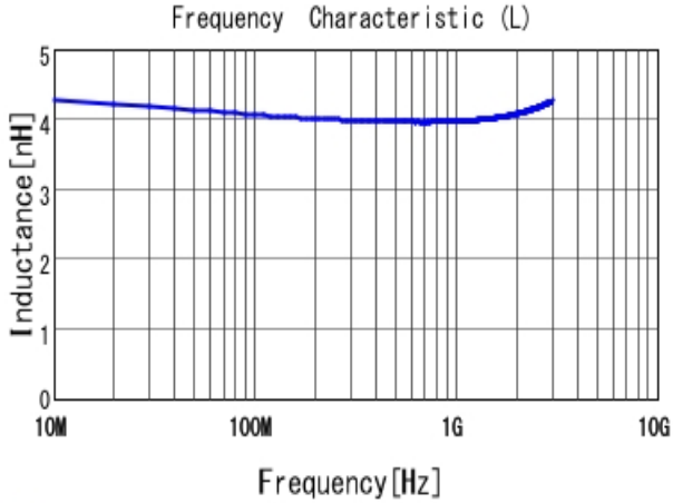
■ LQW15AN4N1C00 L
