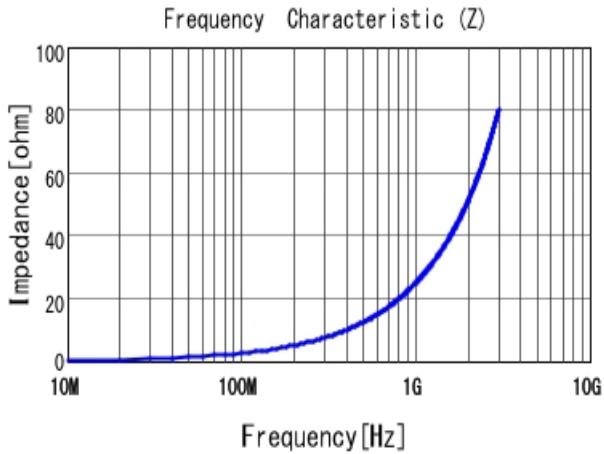
■ LQW15AN4N1C00 |Z|
