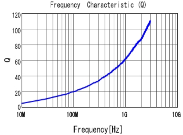
■ LQW15AN4N1C00 Q
