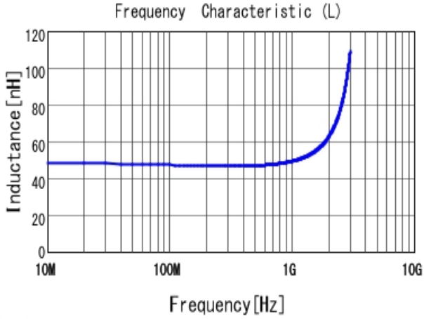
■ LQW15AN47NJ00 L
