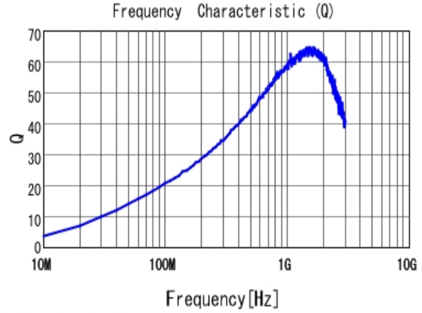
■ LQW15AN47NJ00 Q
