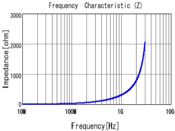
■ LQW15AN47NJ00 |Z|
