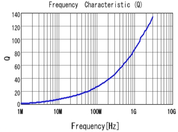
■ LQW15AN3N9G8Z Q
