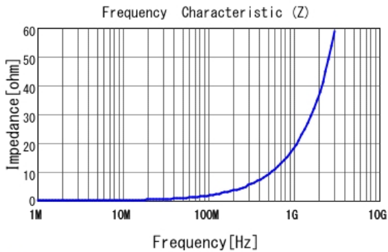
■ LQW15AN3N0C80 |Z|
