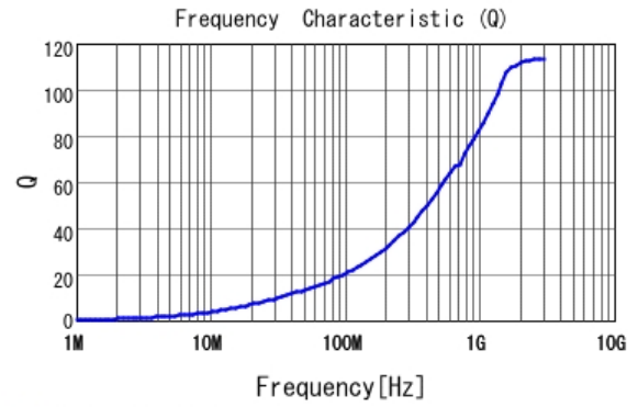
■ LQW15AN3N0C80 Q
