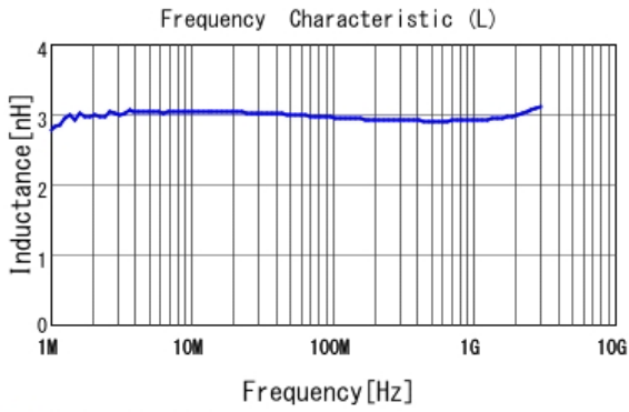
■ LQW15AN3N0C80 L
