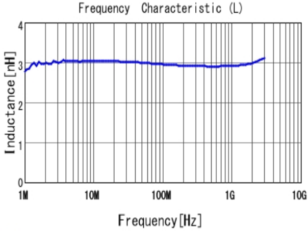
■ LQW15AN3N0B80 L
