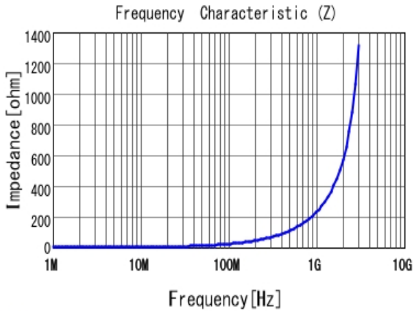
■ LQW15AN36NG80 |Z|
