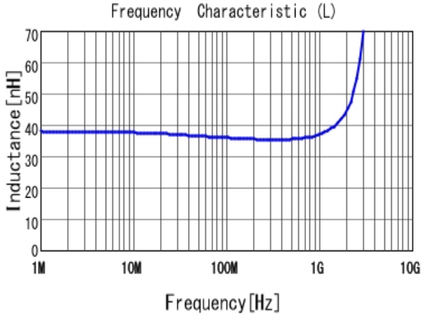
■ LQW15AN36NG80 L
