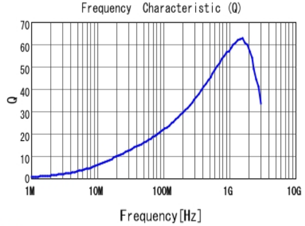
■ LQW15AN36NG80 Q
