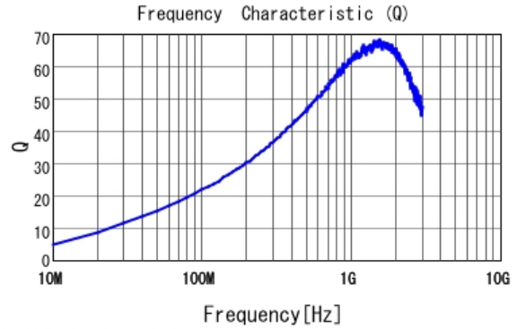
■ LQW15AN36NG00 Q
