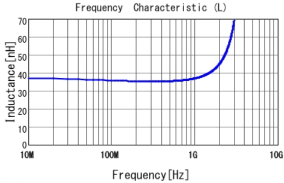
■ LQW15AN36NG00 L
