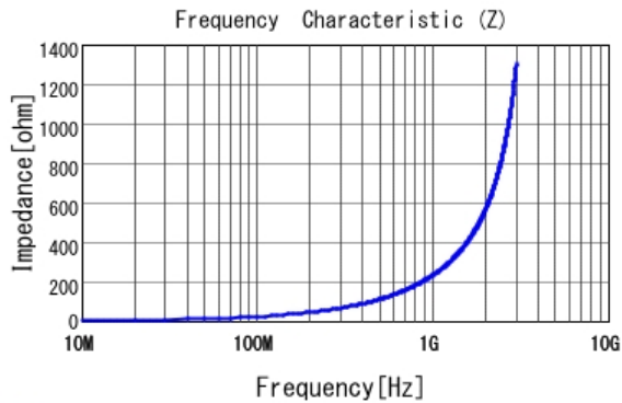
■ LQW15AN36NG00 |Z|
