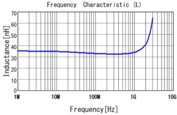
■ LQW15AN33NG80 L
