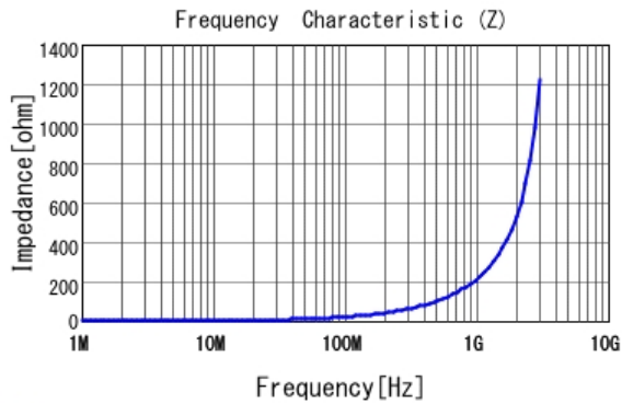
■ LQW15AN33NG80 |Z|
