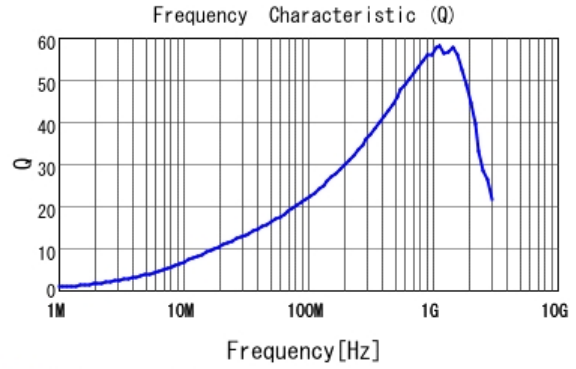
■ LQW15AN33NG80 Q
