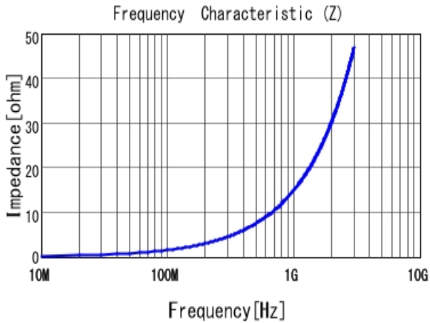
■ LQW15AN2N5C00 |Z|
