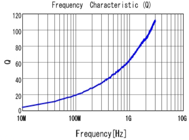
■ LQW15AN2N5C00 Q
