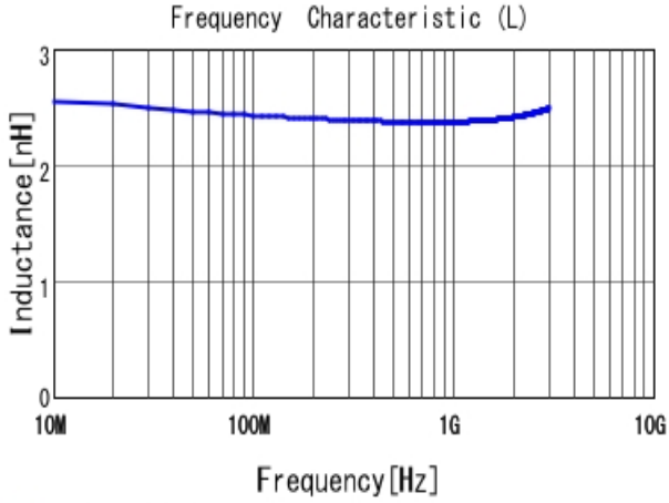
■ LQW15AN2N5C00 L
