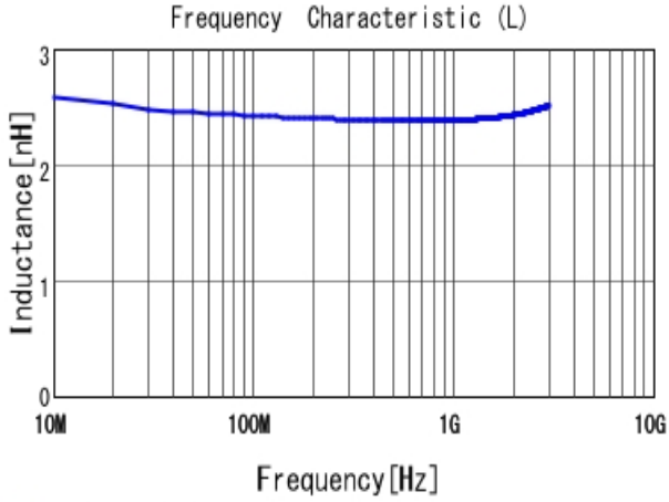
■ LQW15AN2N4D10 L
