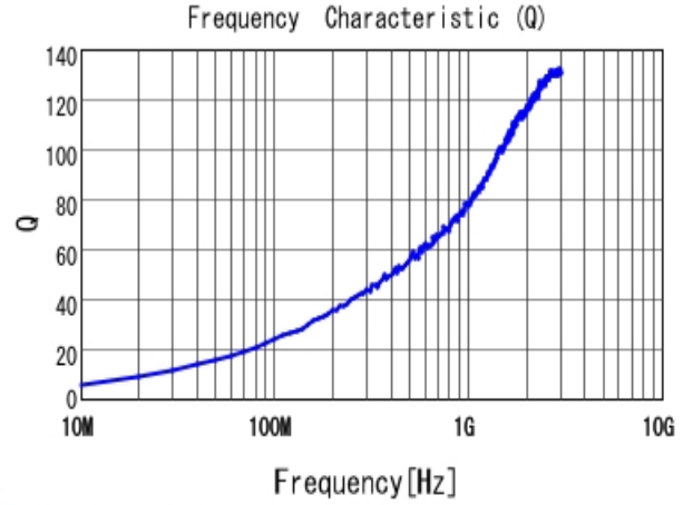
■ LQW15AN2N4D10 Q
