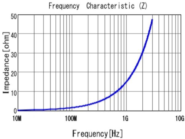
■ LQW15AN2N4D10 |Z|
