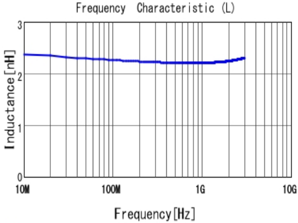
■ LQW15AN2N4C00 L
