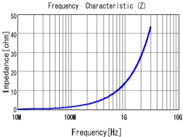
■ LQW15AN2N4C00 |Z|
