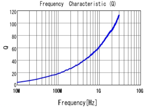
■ LQW15AN2N4C00 Q
