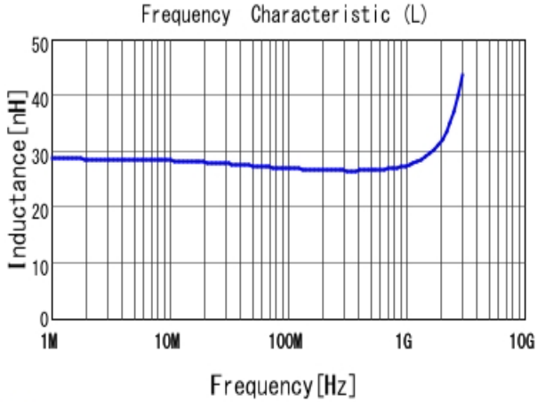
■ LQW15AN27NG80 L
