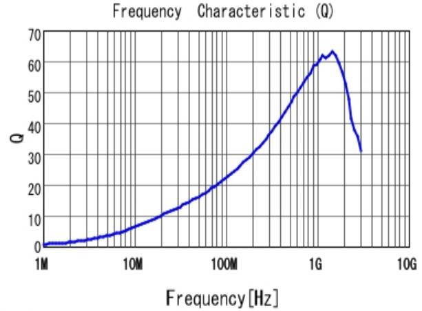
■ LQW15AN27NG80 Q
