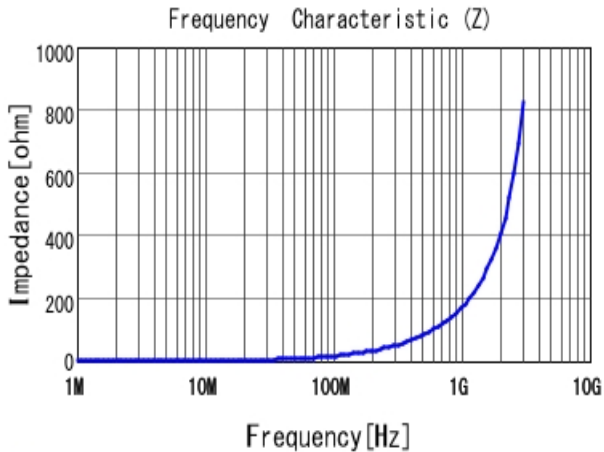
■ LQW15AN27NG80 |Z|
