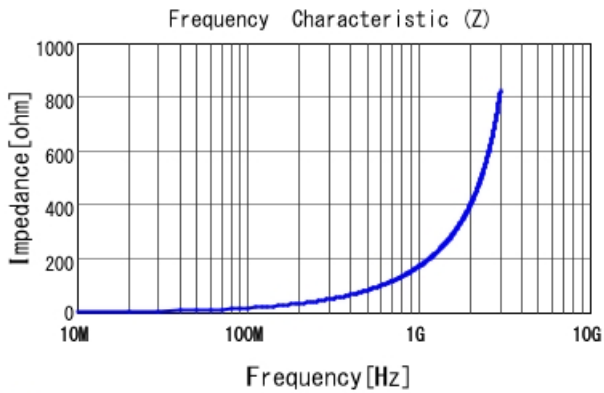
■ LQW15AN27NG00 |Z|
