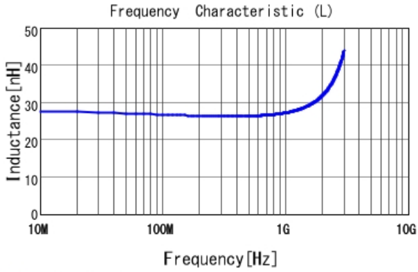
■ LQW15AN27NG00 L
