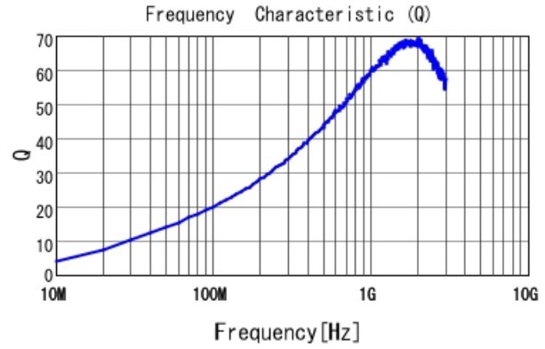
■ LQW15AN27NG00 Q
