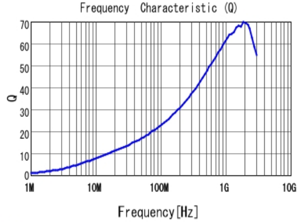
■ LQW15AN22NG80 Q
