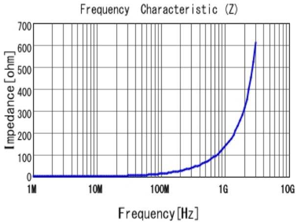
■ LQW15AN22NG80 |Z|
