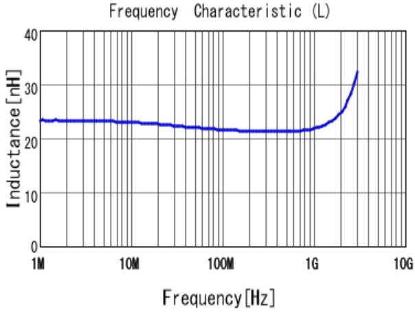
■ LQW15AN22NG80 L
