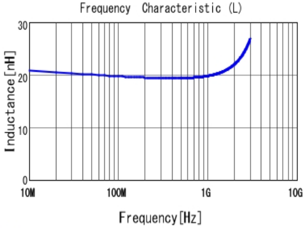
■ LQW15AN20NJ00 L
