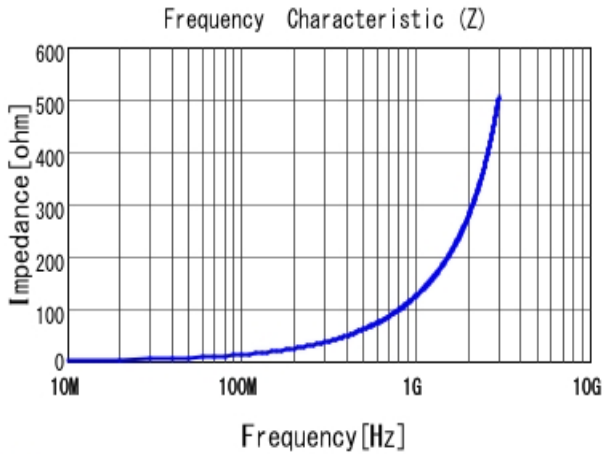
■ LQW15AN20NJ00 |Z|
