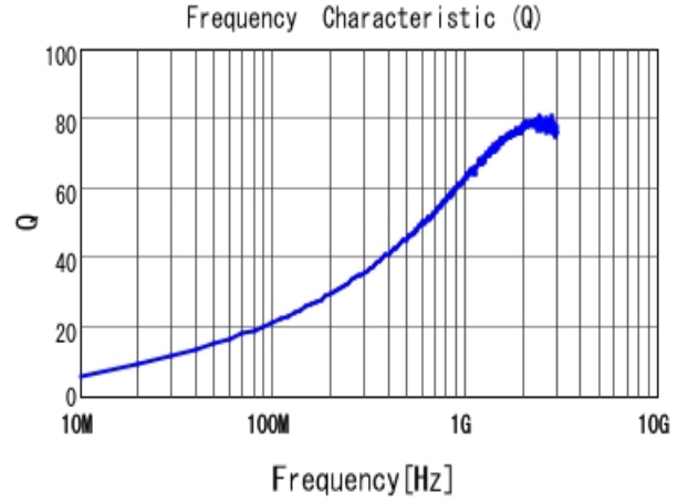
■ LQW15AN20NJ00 Q
