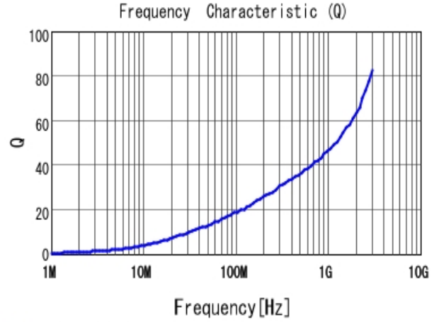
■ LQW15AN1N5C80 Q
