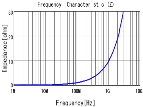
■ LQW15AN1N5C80 |Z|
