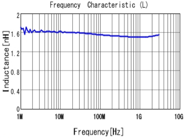
■ LQW15AN1N5C80 L
