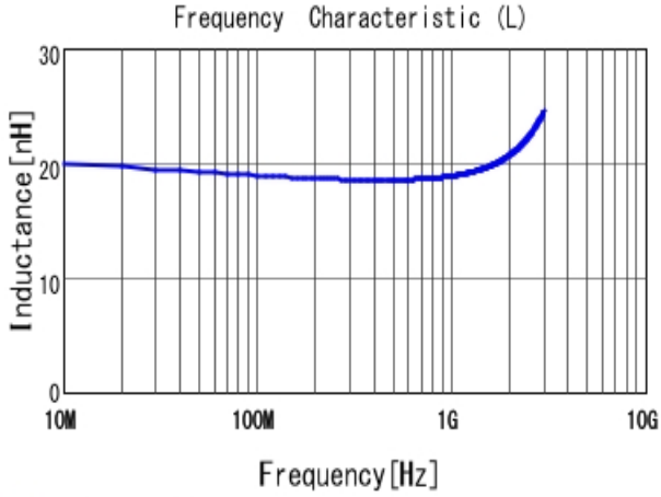
■ LQW15AN19NJ00 L
