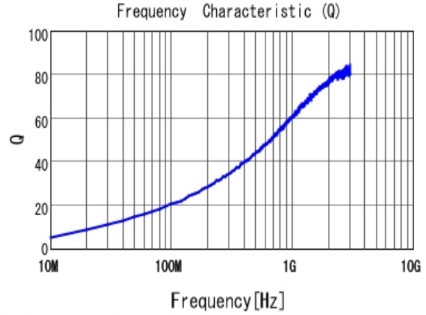
■ LQW15AN19NJ00 Q
