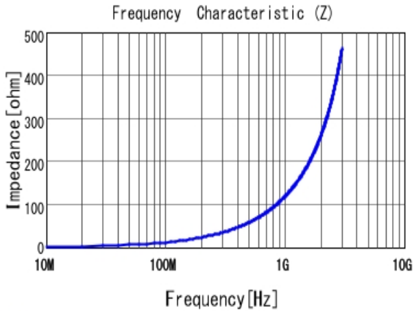
■ LQW15AN19NJ00 |Z|
