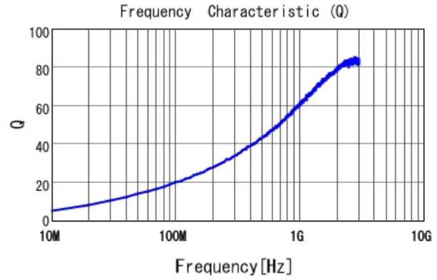
■ LQW15AN16NJ00 Q
