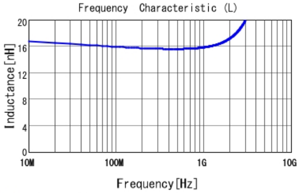
■ LQW15AN16NJ00 L
