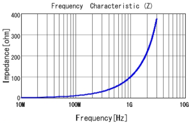
■ LQW15AN16NJ00 |Z|
