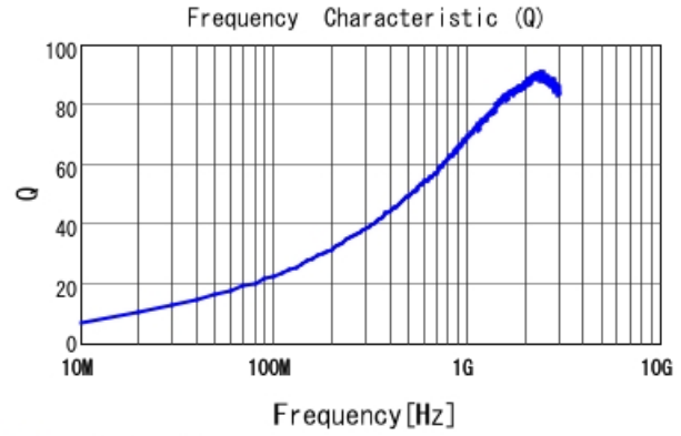
■ LQW15AN15NH00 Q
