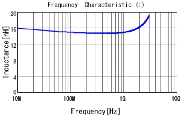
■ LQW15AN15NH00 L
