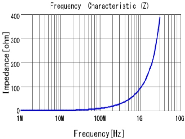
■ LQW15AN15NG8Z |Z|
