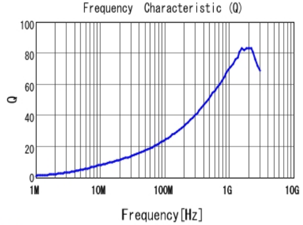
■ LQW15AN15NG8Z Q
