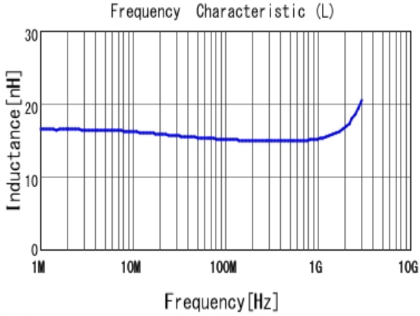
■ LQW15AN15NG8Z L
