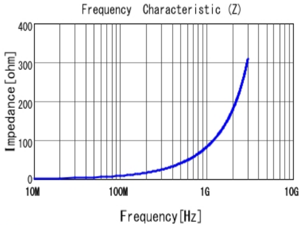
■ LQW15AN13NJ00 |Z|
