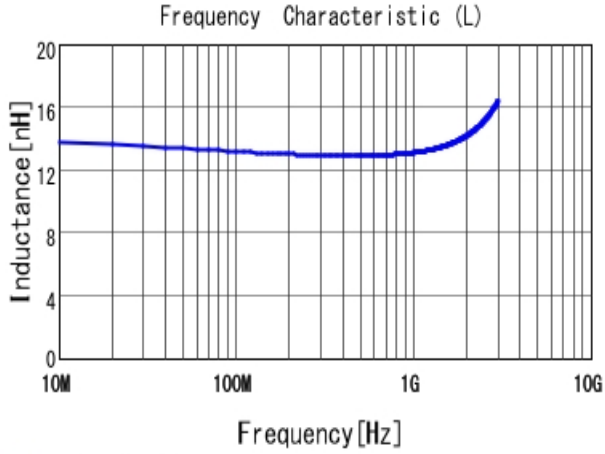
■ LQW15AN13NJ00 L
