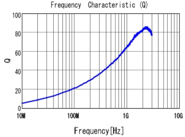
■ LQW15AN13NJ00 Q
