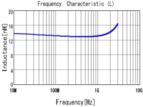
■ LQW15AN13NH00 L
