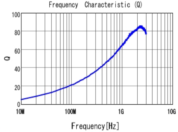
■ LQW15AN13NH00 Q
