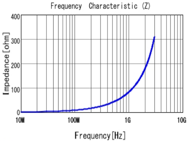
■ LQW15AN13NG00 |Z|
