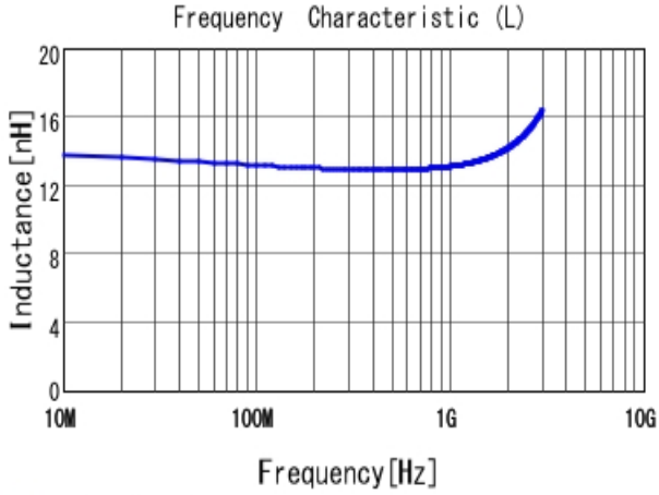
■ LQW15AN13NG00 L
