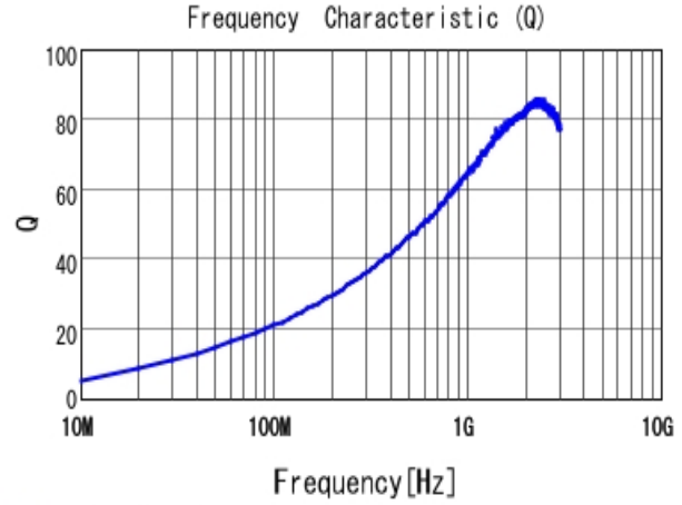
■ LQW15AN13NG00 Q
