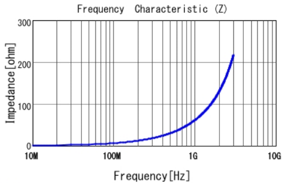
■ LQW15AN10NJ00 |Z|
