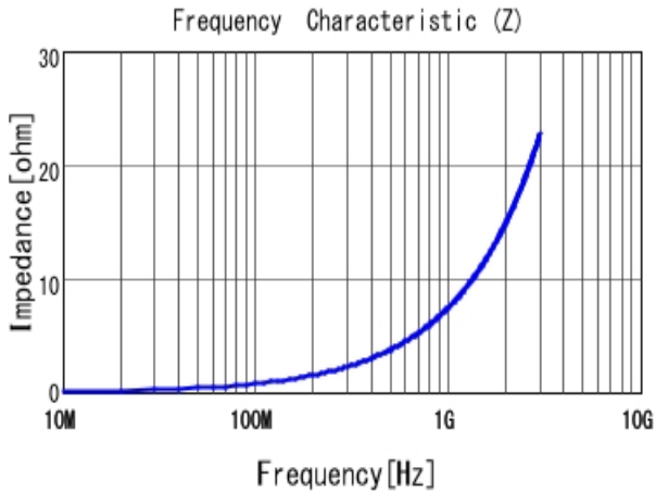
■ LQP15MN1N2B02 |Z|
